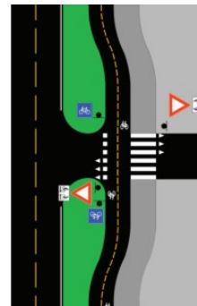
Figur 51: Kryssing mellom veg og sykkelveg med fortau der kryssende trafikk skal vike for syklende. faksimile V122 SVV.
