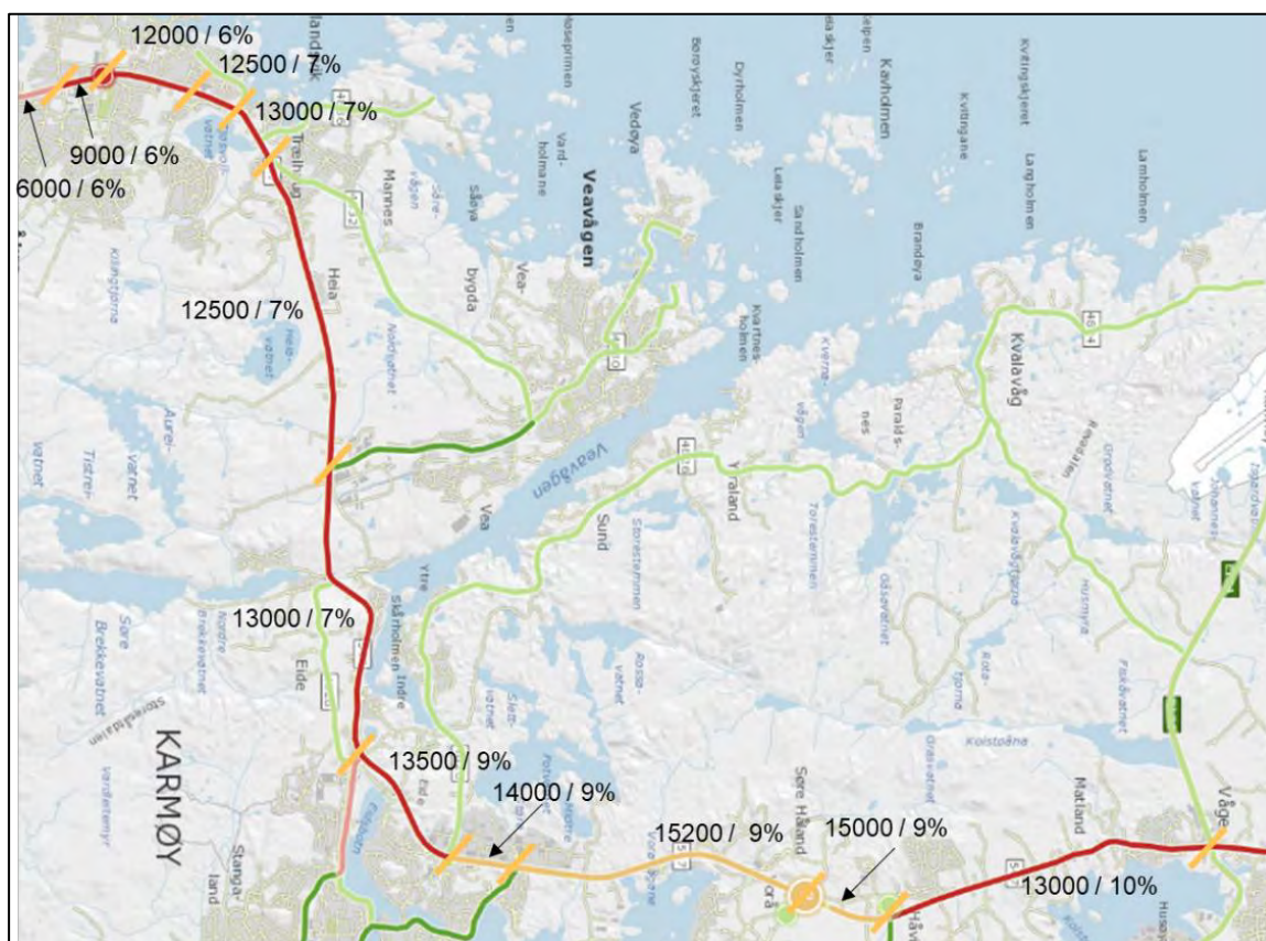
Figur 2-16 Trafikkmengder og tungtrafikkandel 2019, Kilde: Vegkart (vegvesen.no)
